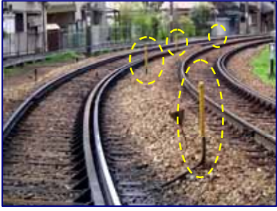
限界支障報知装置 (点線で囲んだ部分が検知柱)
