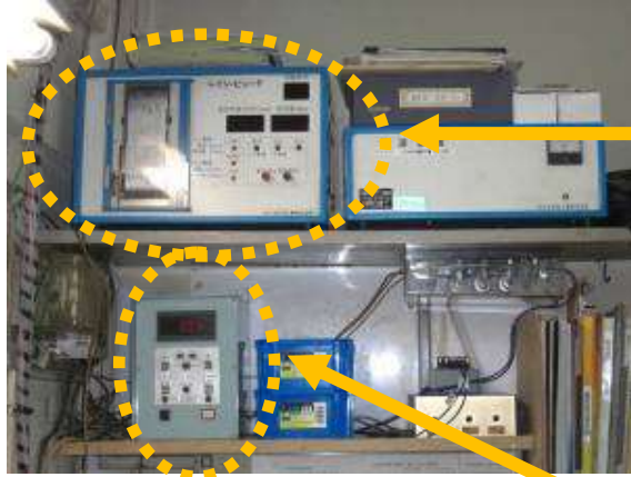
山上駅の雨量監視装置及び風速監視装置
